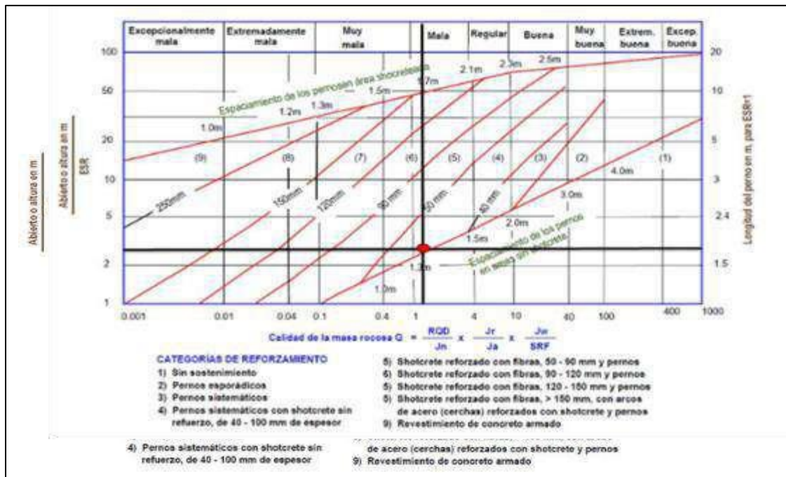
Figura 16. Sostenimiento recomendado para la VN639_10, Nv-4100
