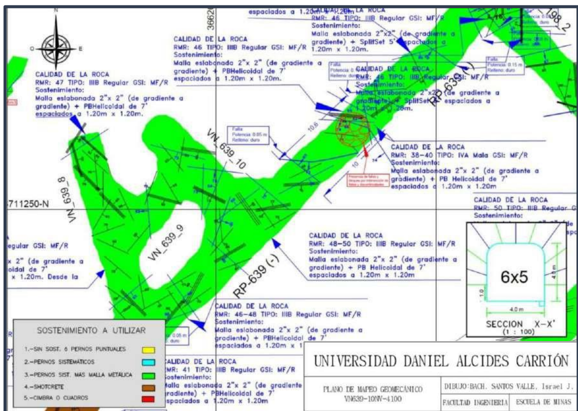
Plano 1. Plano de mapeo geomecanico vn639_10, nv-4100
