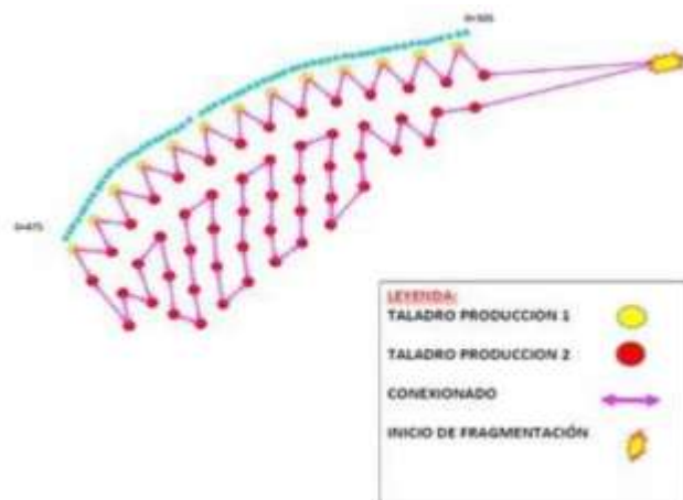
Figura 32. Malla de Perforación y Orden de Salida.
