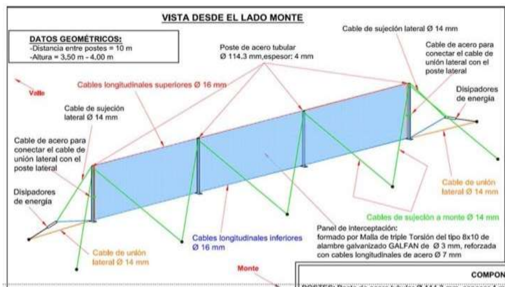
Figura 24. Barrera dinámica situada en los frentes 04 y 05
