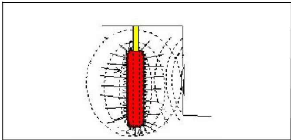
Ilustración 15. Propagación de ondas de choque y esfuerzos
