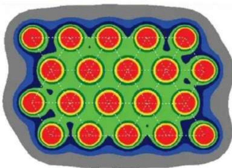
Figura 3. Elaboración de la malla triangular equilátera
