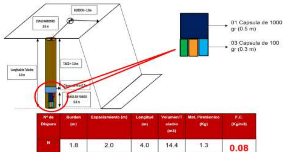
Figura 21. Componente de carga
