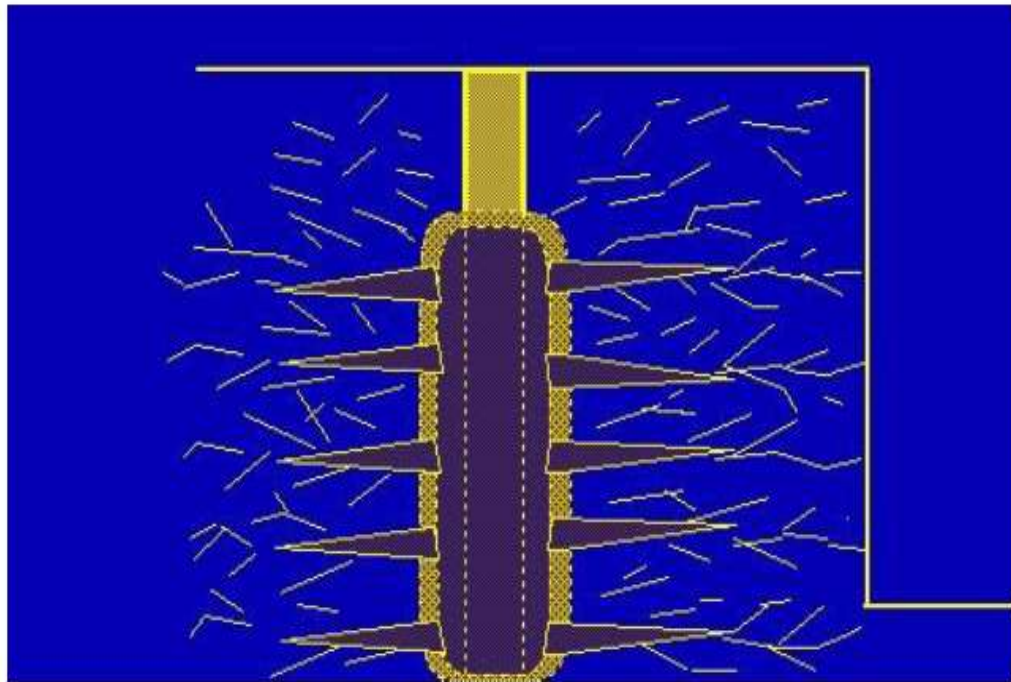
Ilustración 16. Expansión de gases y agrietamiento
