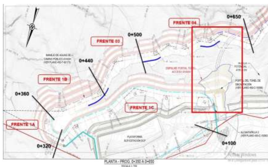
Figura 11. Zona de labor gradual 0 + 350 a 0 + 650
