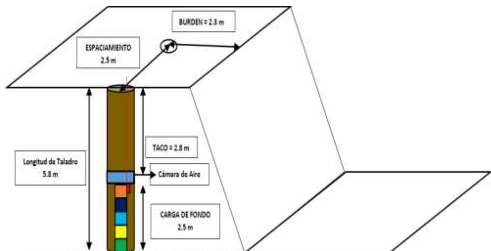
Figura 31. Elemento de Carga Taladros de Producción
