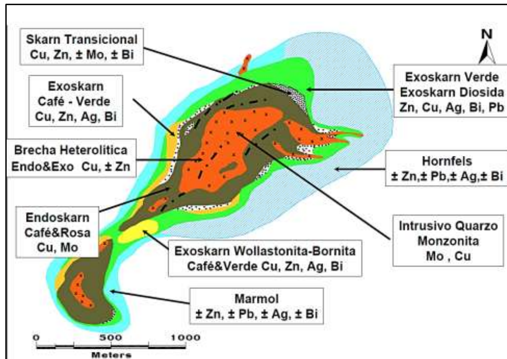
Ilustración 7. Esquema Litológico y Zoneamiento de Antamina
