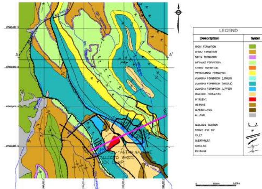
Ilustración 3. Geología Regional del Yacimiento Antamina.
