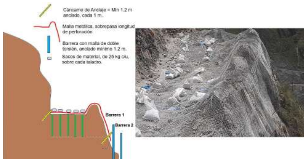
Figura 20. Inspecciones de fragmentación
