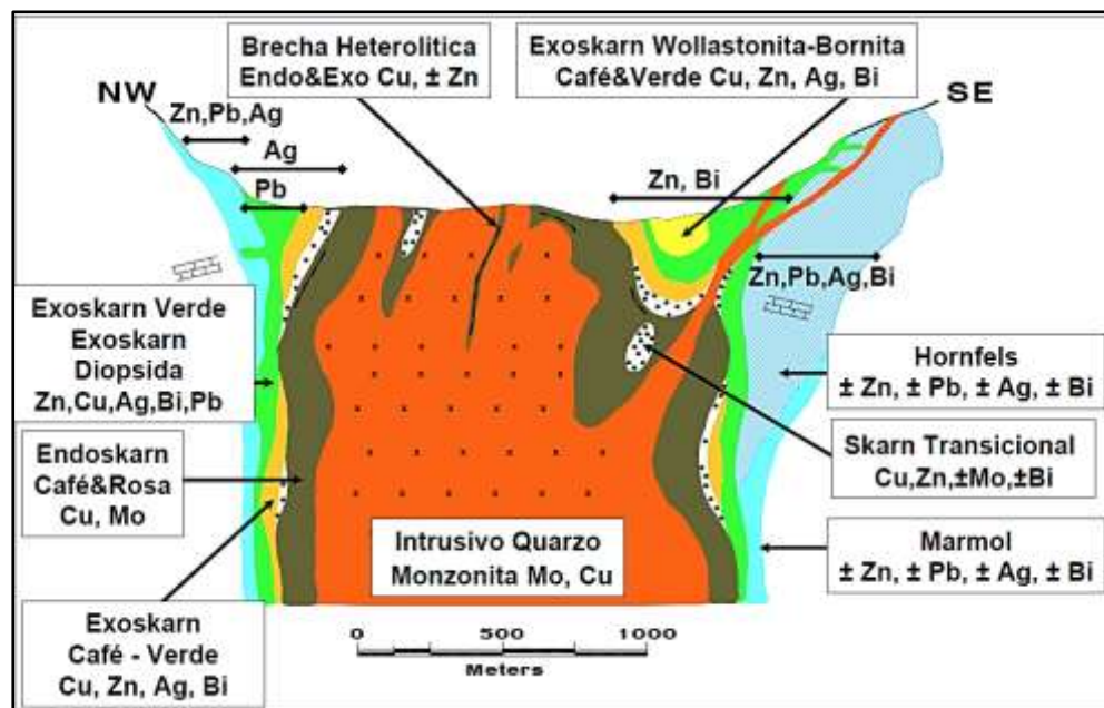
Ilustración 8. Esquema Litológico y Zoneamiento de Antamina
