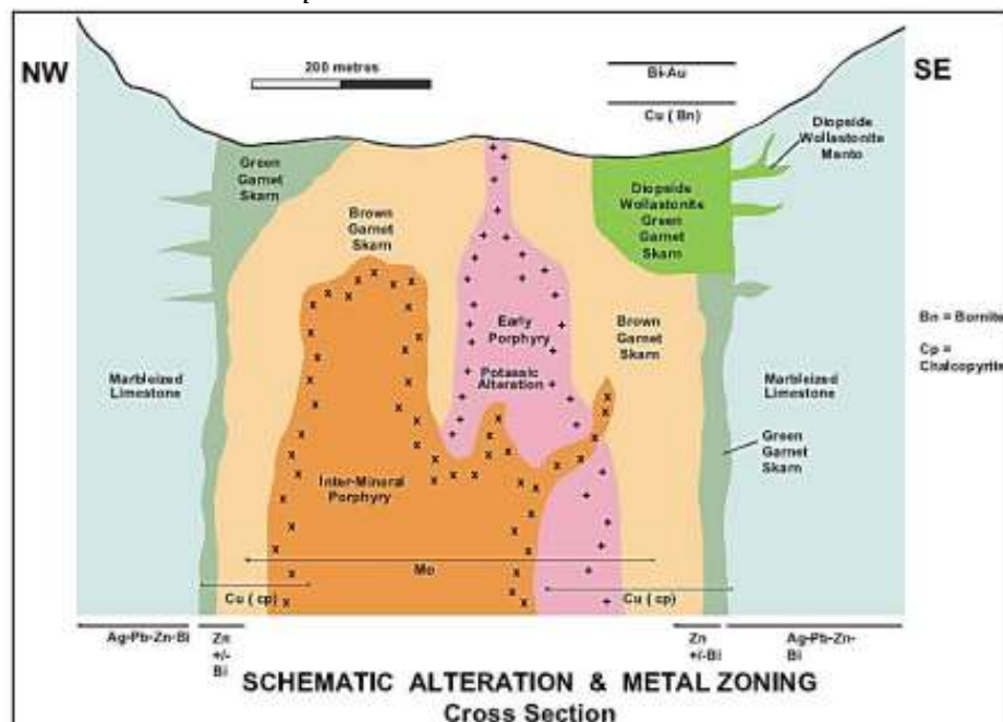
Ilustración 6. Esquema de Alteraciones en sección de Antamina.
