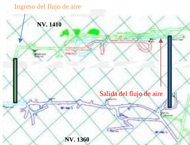
Figura 7. Circuito de ventilación
