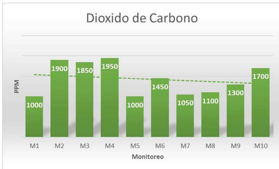
Figura 15. Dióxido de carbono optimizado
