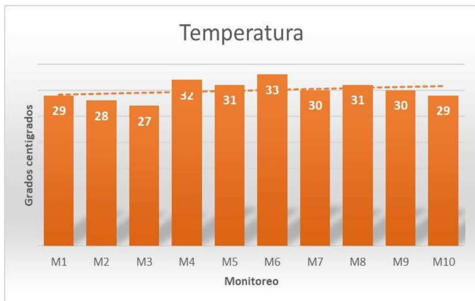
Figura 9. Temperatura inicial
