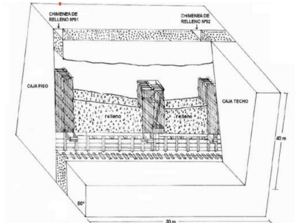
Figura 4. Método de corte y relleno ascendente
