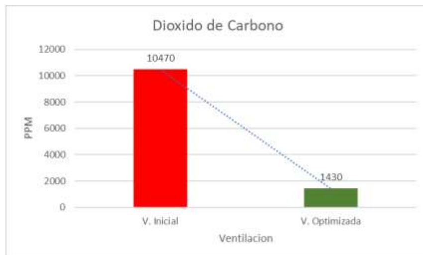
Figura 19. Relación de ventilación en dióxido de carbono
