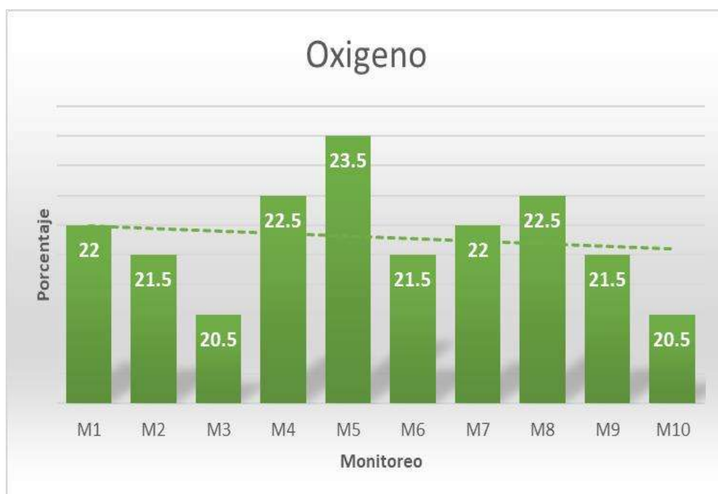
Figura 14. Porcentaje de oxígeno optimizado
