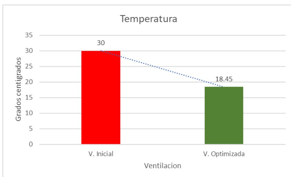
Figura 17. Relación de la temperatura
