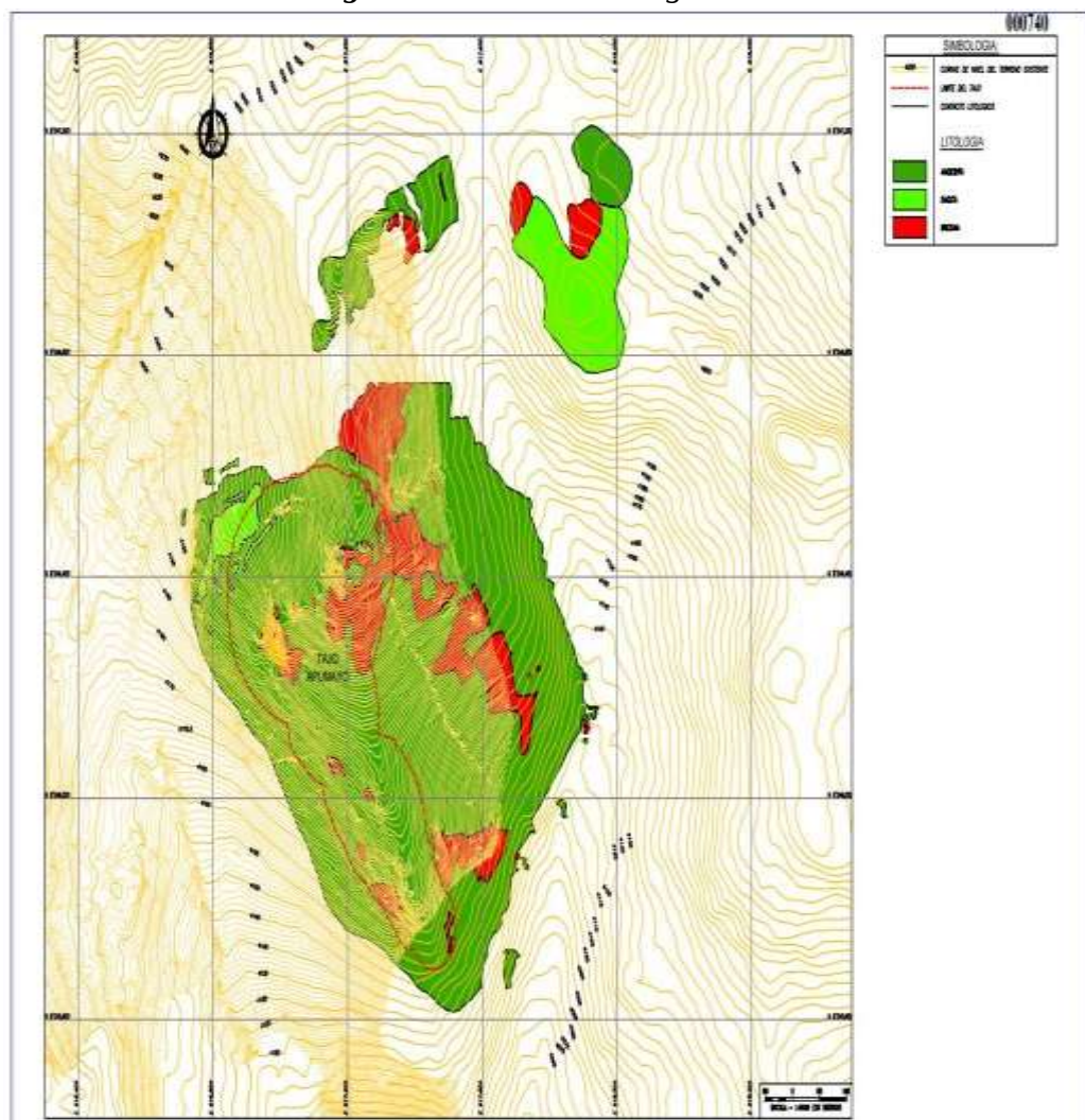
Figura 3. Plano de Geología Local
