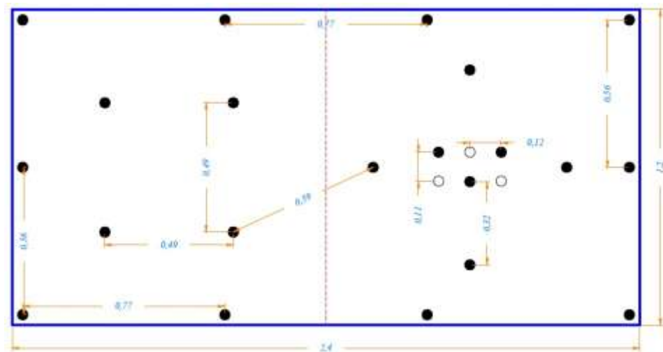
Figura 6. Malla de perforación - Chimenea 4x8
