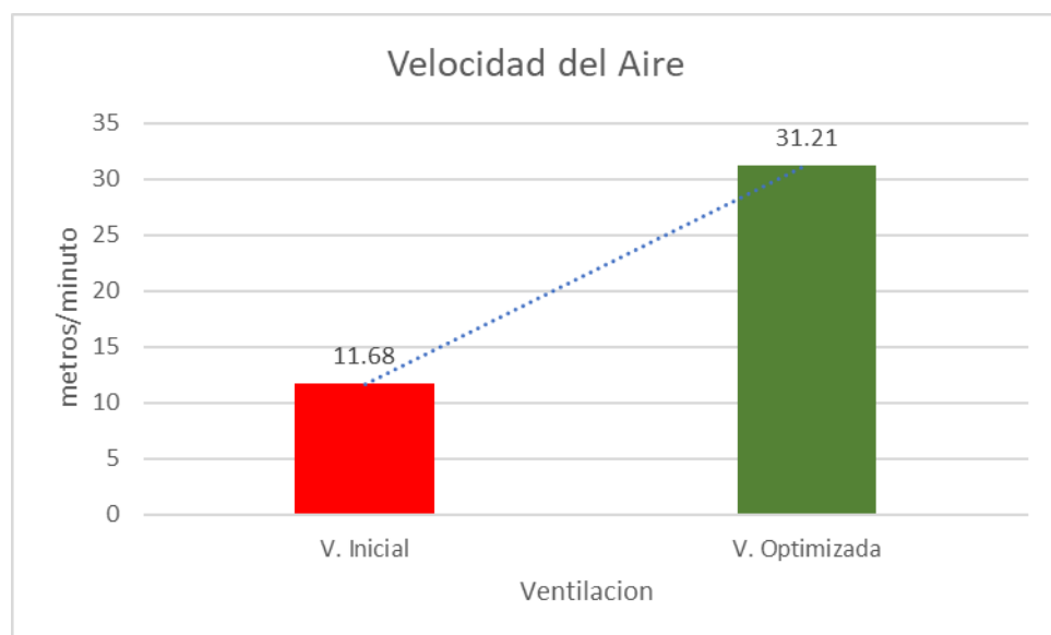
Figura 16. Relación de la velocidad de aire
