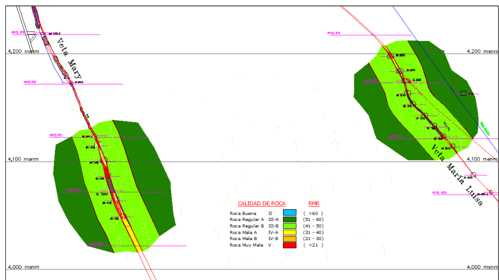
Ilustración 16. Ejemplo de la Zonificación Geomecánica
