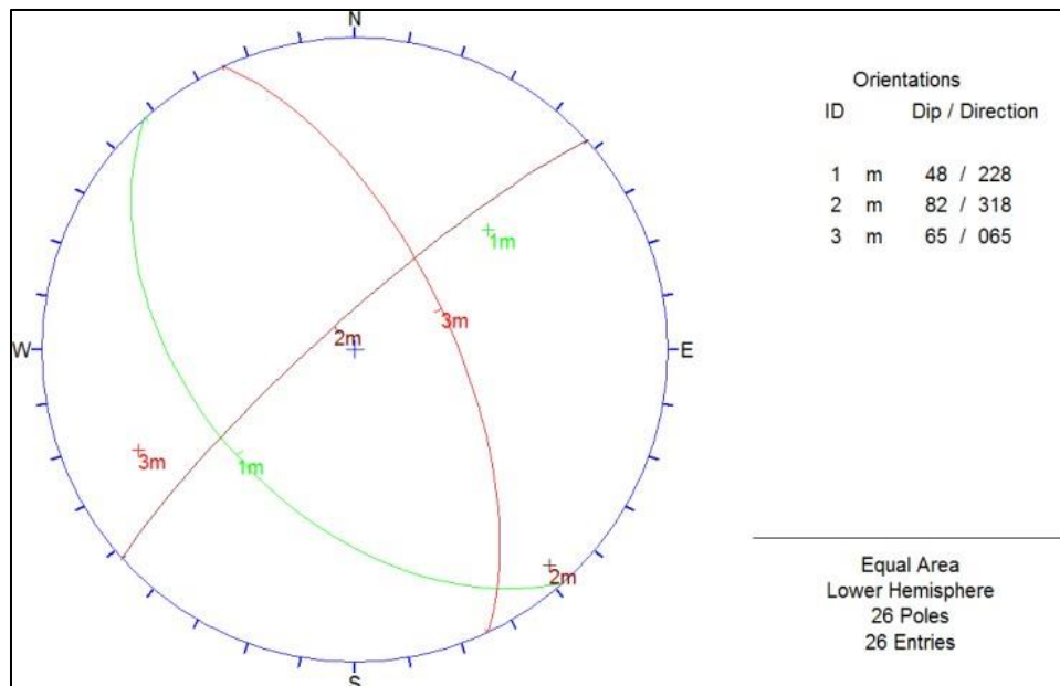
Ilustración 14. Cuerpo Huaripampa - Diagrama Estereográfico de Planos Principales del Compósito de Discontinuidades.
