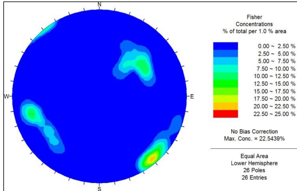
Ilustración 13. Cuerpo Huaripampa - Estereográfico de Contornos del Compósito de Discontinuidades.
