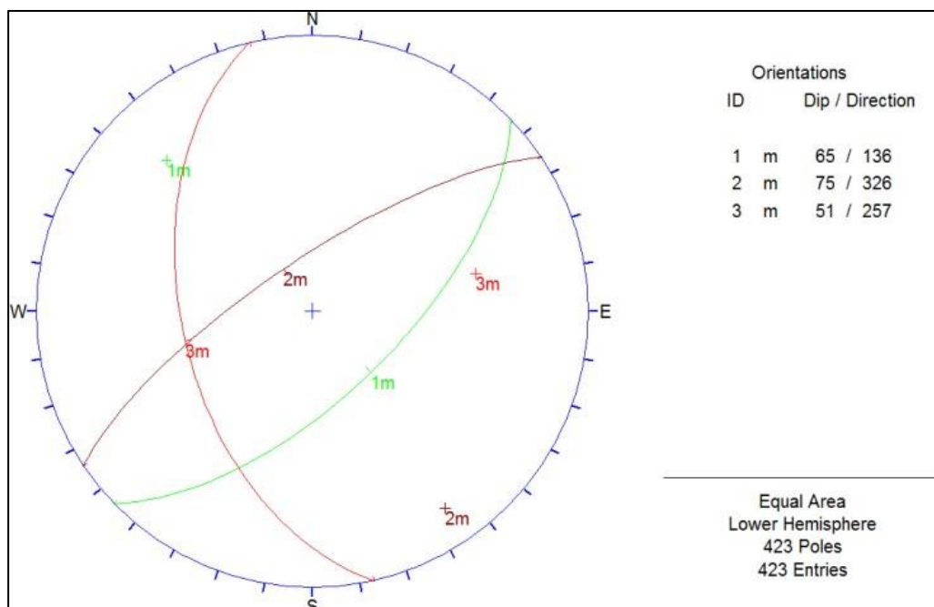
Ilustración 10. Veta Maria Luisa - Estereográfico de Contornos del Compósito de Discontinuidades.
