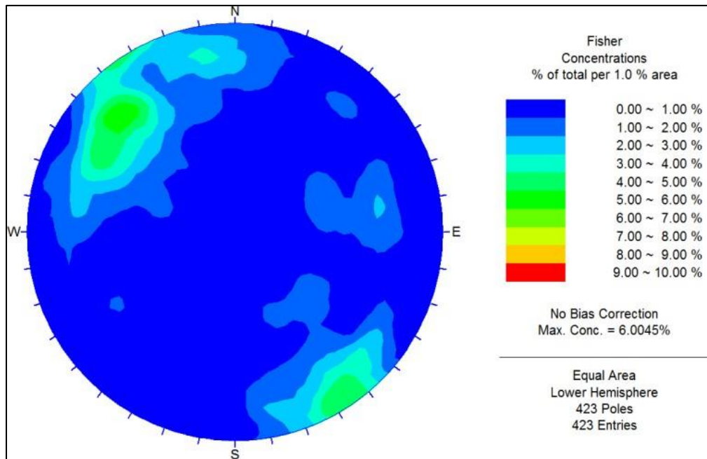
Ilustración 11. Veta Maria Luisa - Diagrama Estereográfico de Planos Principales del Compósito de Discontinuidades.
