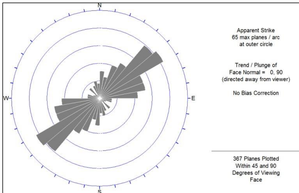
Ilustración 12. Veta Maria Luisa - Diagrama de Roseta del Compósito de Discontinuidades.
