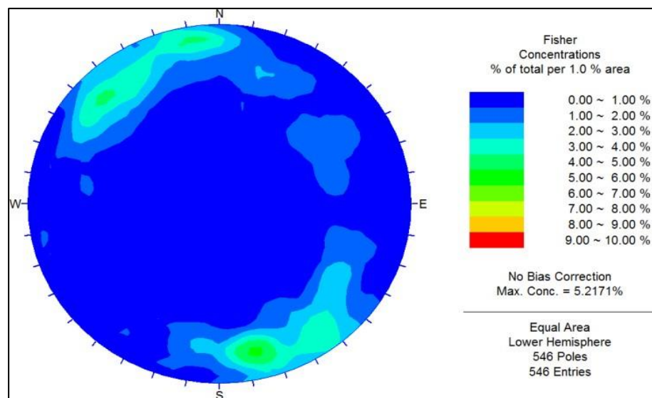
Ilustración 8. Veta Mary - Diagrama Estereográfico de planos Principales del Compósito de Discontinuidades.
