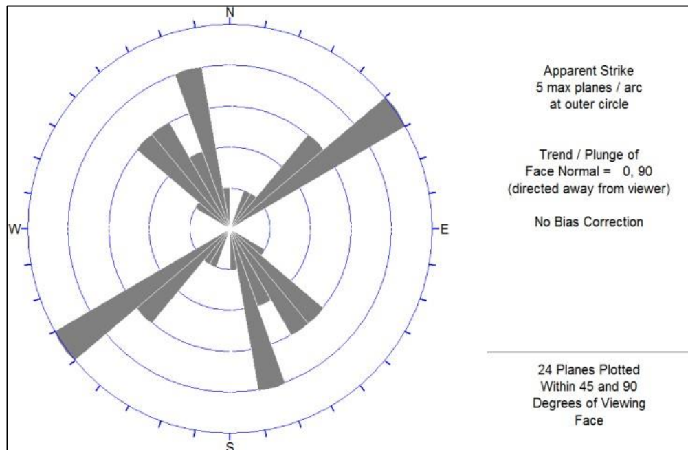
Ilustración 15. Cuerpo Huaripamapa - Diagrama de Roseta del Compósito de Discontinuidades.
