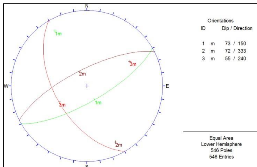
Ilustración 8. Veta Mary - Diagrama Estereográfico de planos Principales del Compósito de Discontinuidades.
