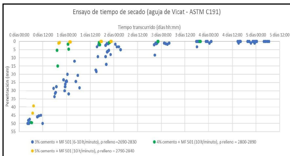
Ilustración 28. Ensayo de tiempo de secado con herramienta vicat
