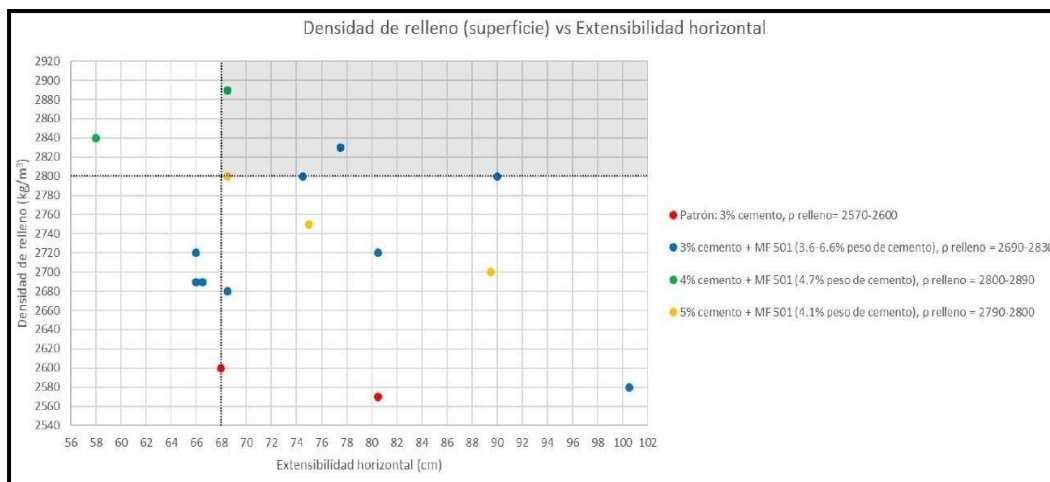
Ilustración 26. Densidad del Relleno Hidráulico Vs Extensibilidad Horizontal
